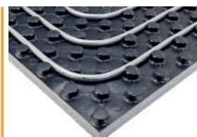
Sujeción segura del tubo con paso a múltiplos de 50 mm.
