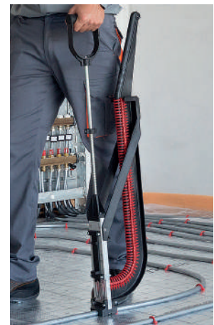
Grapadora específica para grapa 3D.
