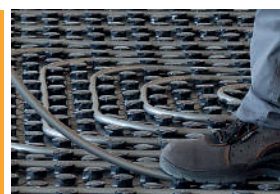
Sencilla y cómoda colocación del tubo.
